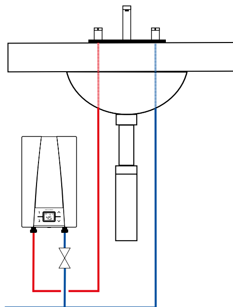
Прямое подключение: Водоснабжение одной водоразборной точки
