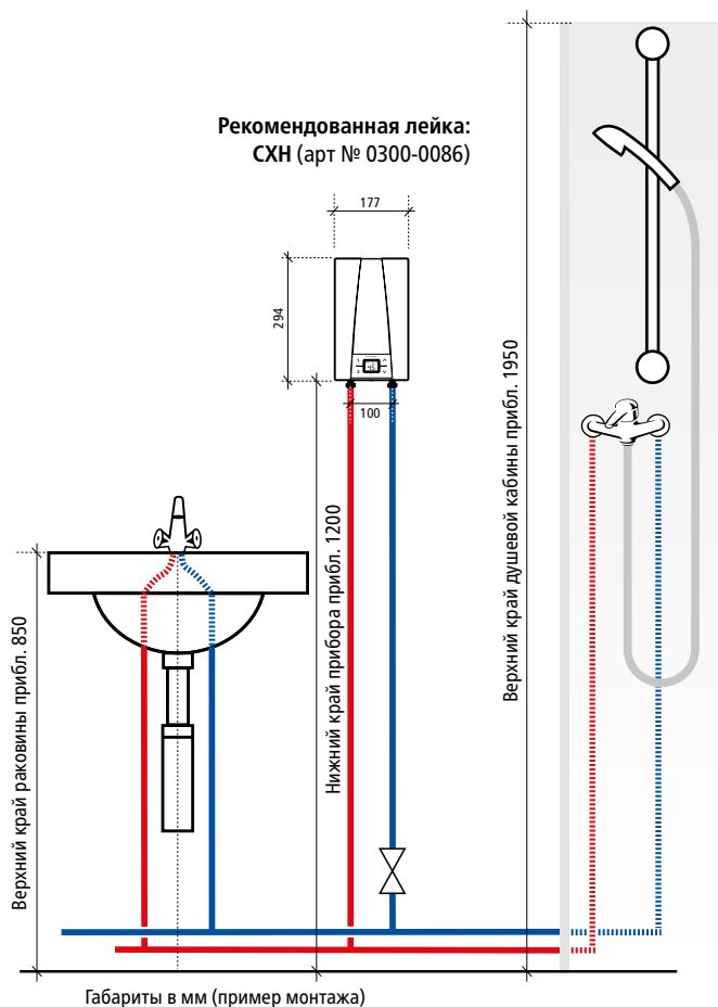
Прямое подключение: Водоснабжение нескольких водоразборных точек
